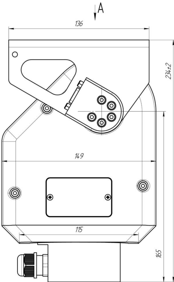
Рис. Б.2 Габаритные и установочные размеры двухканального исполнения ОПУ
