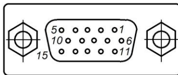
Нумерация контактов гнезда DHB-15
